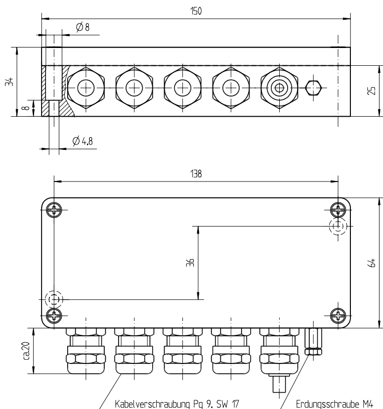
Abbildung 2, Maßbild XKC 251
