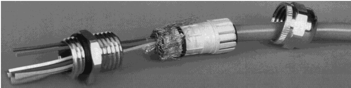
Abbildung 5, Kabelmontage
