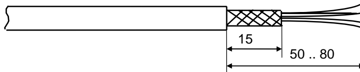
Abbildung 4, Absetzen des Kabels
