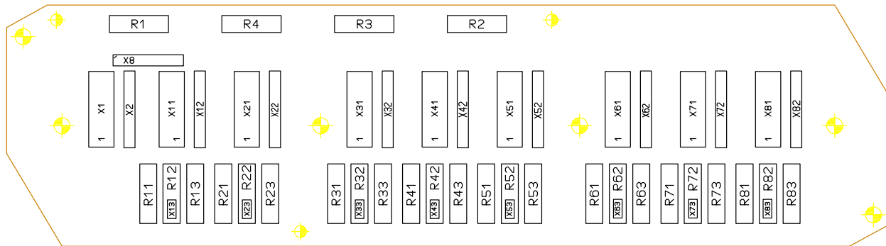
Abbildung 8, Leiterplatte XKC 256
