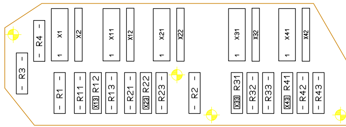
Abbildung 7, Leiterplatte XKC 251
