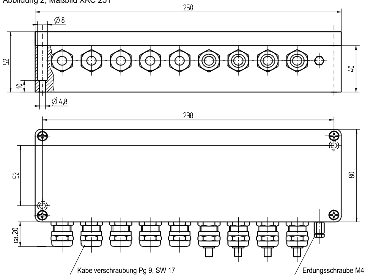
Abbildung 3, Maßbild XKC 256
